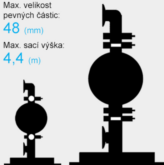
Porovnání standardního čerpadla s kulíovým ventilem a čerpadla se zpětnou klapkou.
