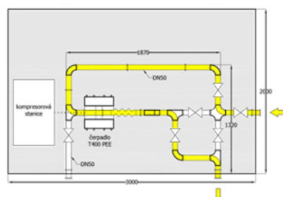
(Schéma provozu přečerpávací stanice)
